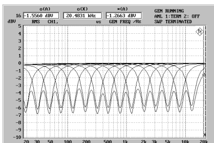
GE230 Response with alternate bands set to minimum Respuesta con bandas alternadas al mínimo
