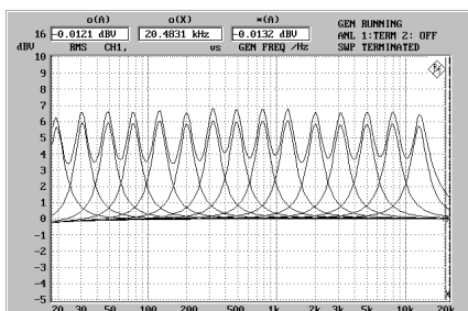
GE230 Response with alternate bands set to maximum Respuesta con bandas alternadas al máximo
